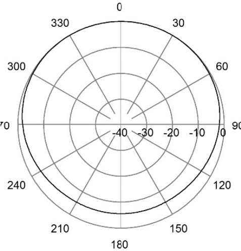
H-Plane | 459 MHz
