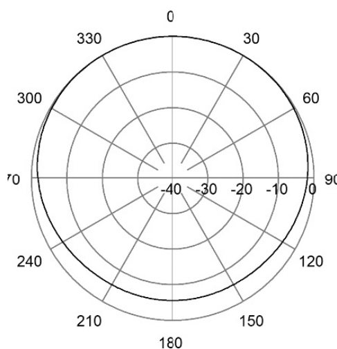
H-Plane | 445 MHz
