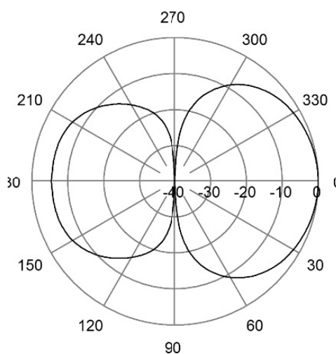
E-Plane | 445 MHz
